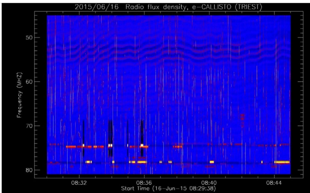
Fig. 4: Scariche atmosferiche visibili nello spettro 45-80 MHz
