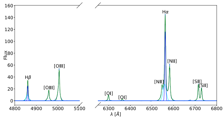
Figure D2. IRAS 23128–5919.
