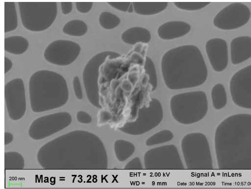
Fig. 4. Particle D08C_017.
