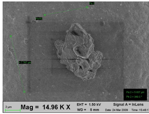
Fig. 3. Particle D08C_006.
