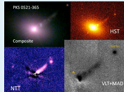
Fig. 1 Multiband images of PKS 0521-365
