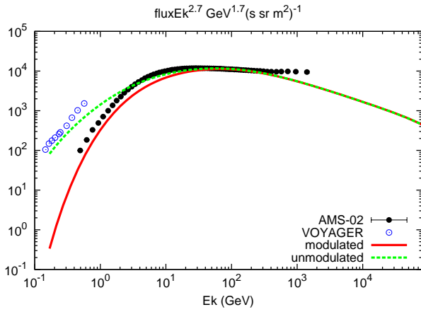
(b) Model-B: CR spectrum.
