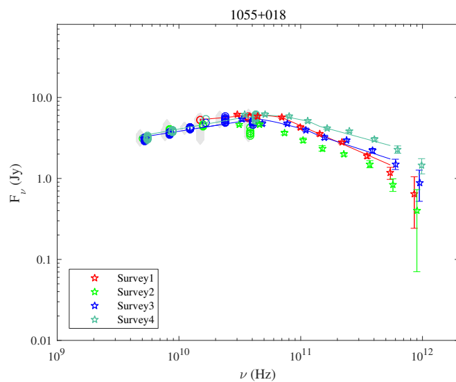
Fig. A.50. 1055+018.
