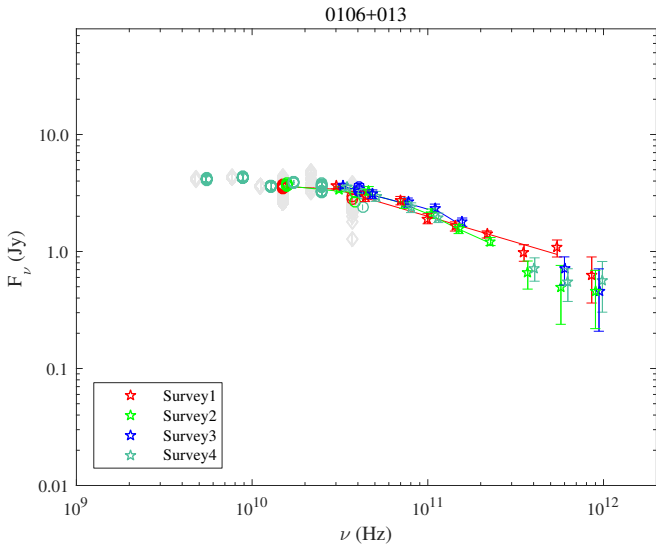
Fig. A.5. 0106+013.
