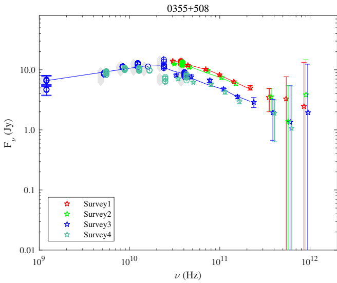
Fig. A.19. 0355+508.
