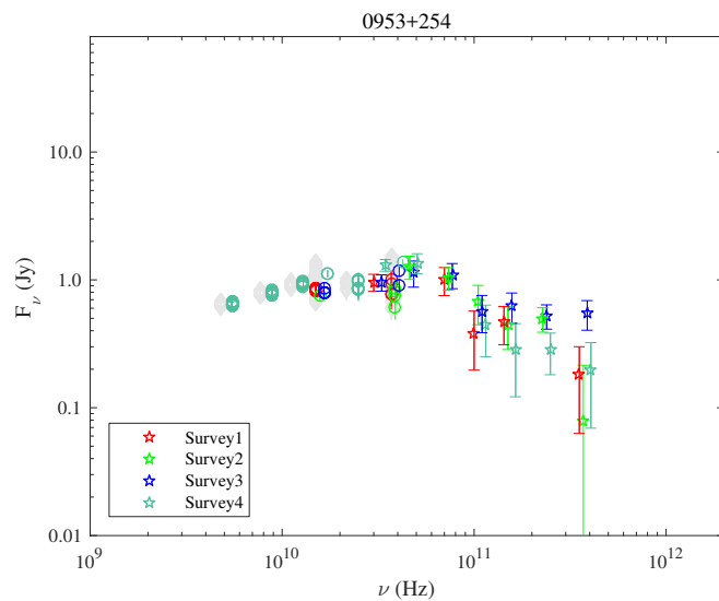
Fig. A.46. 0953+254.
