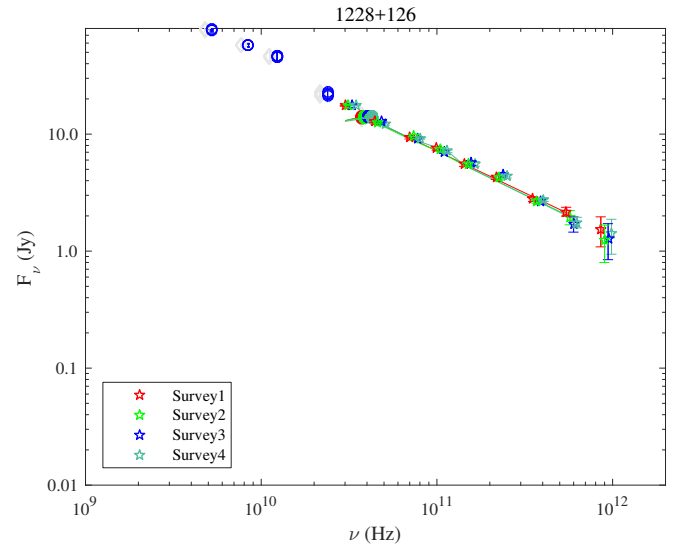
Fig. A.58. 1228+126.
