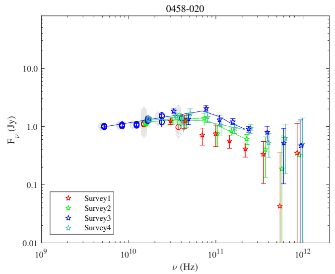
Fig. A.24. 0458-020.
