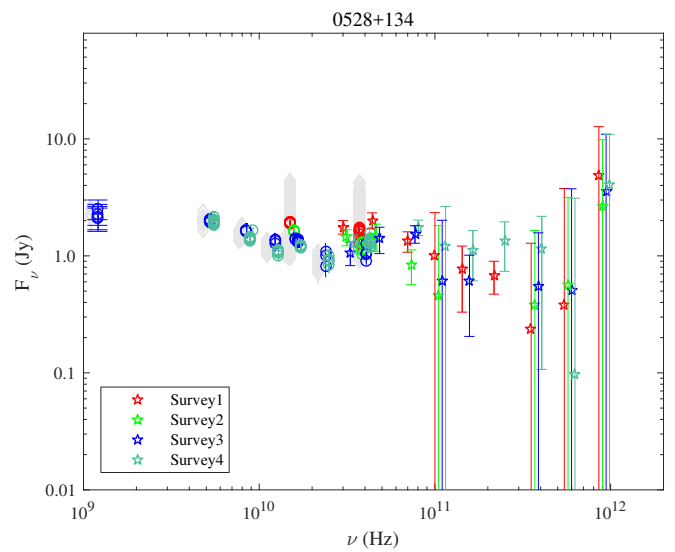
Fig. A.26. 0528+134.
