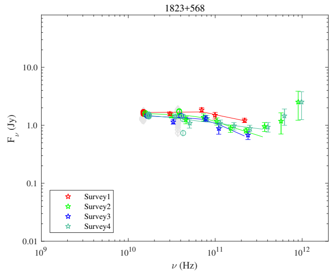
Fig. A.80. 1823+568.
