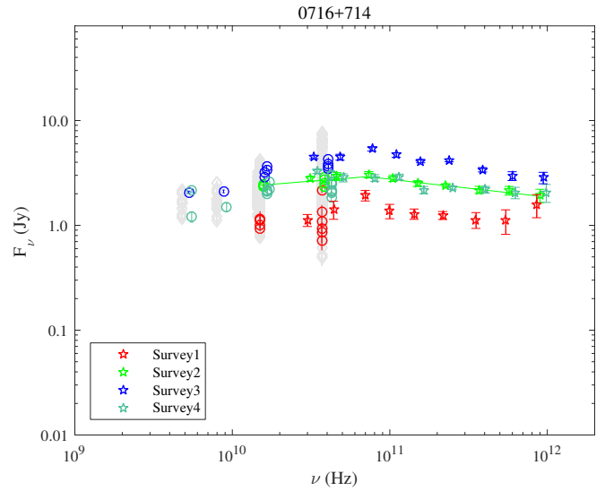
Fig. A.30. 0716+714.
