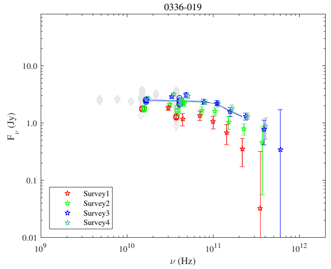
Fig. A.18. 0336-019.
