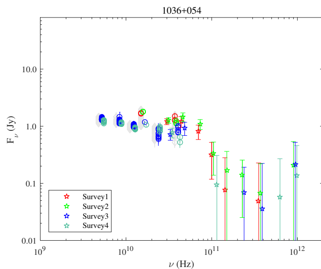
Fig. A.48. 1036+054.
