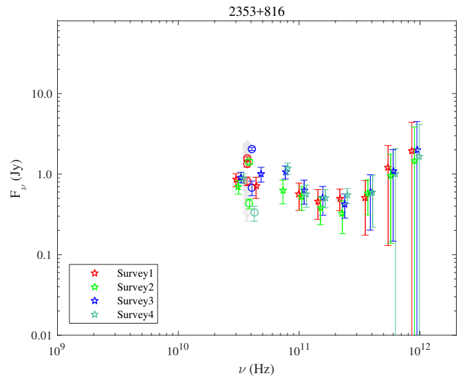
Fig. A.104. 2353+816.
