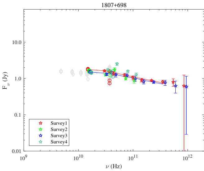
Fig. A.79. 1807+698.
