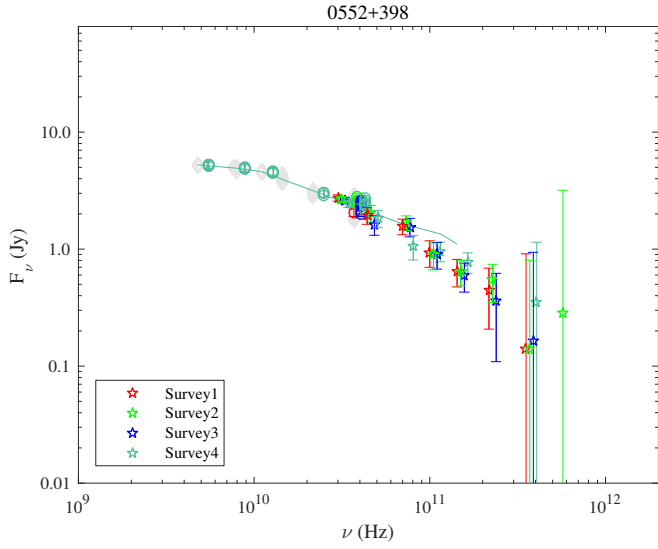
Fig. A.27. 0552+398.
