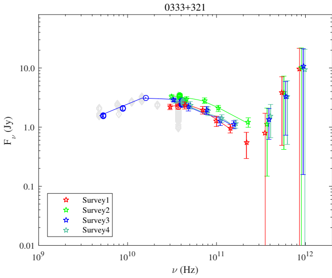
Fig. A.17. 0333+321.
