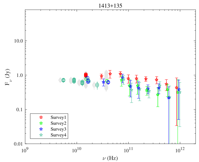
Fig. A.62. 1413+135.
