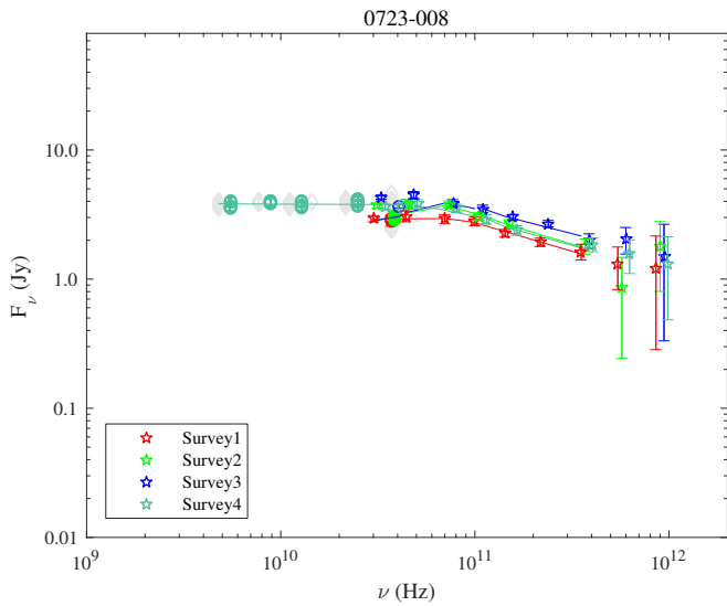
Fig. A.31. 0723-008.
