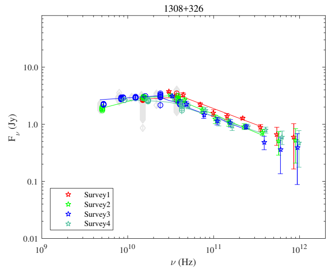
Fig. A.60. 1308+326.
