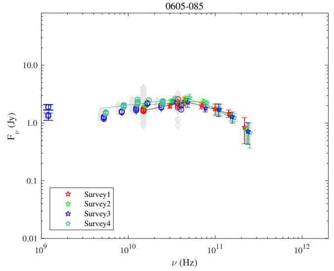
Fig. A.28. 0605-085.
