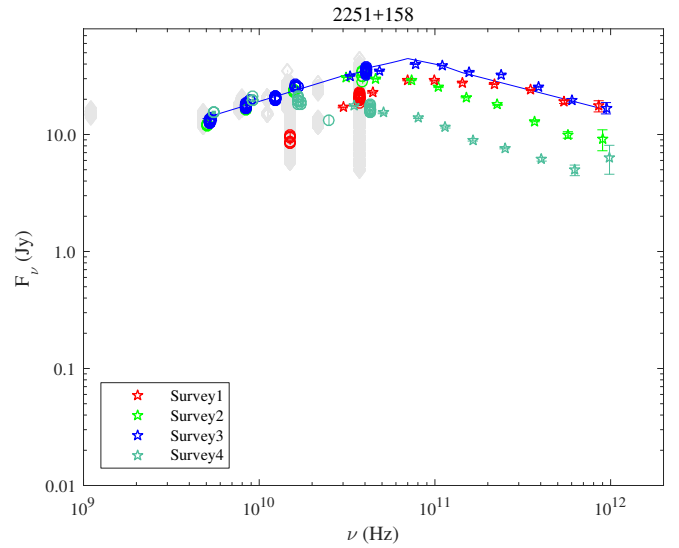
Fig. A.102. 2251+158.
