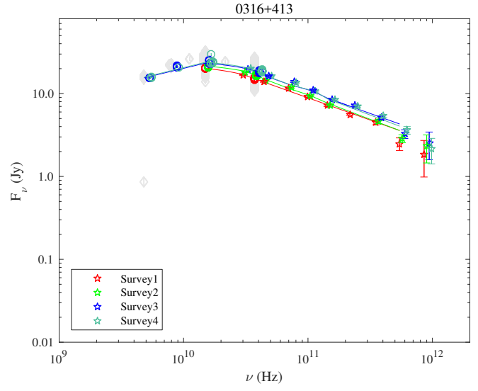
Fig. A.16. 0316+413.
