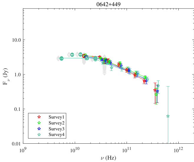
Fig. A.29. 0642+449.
