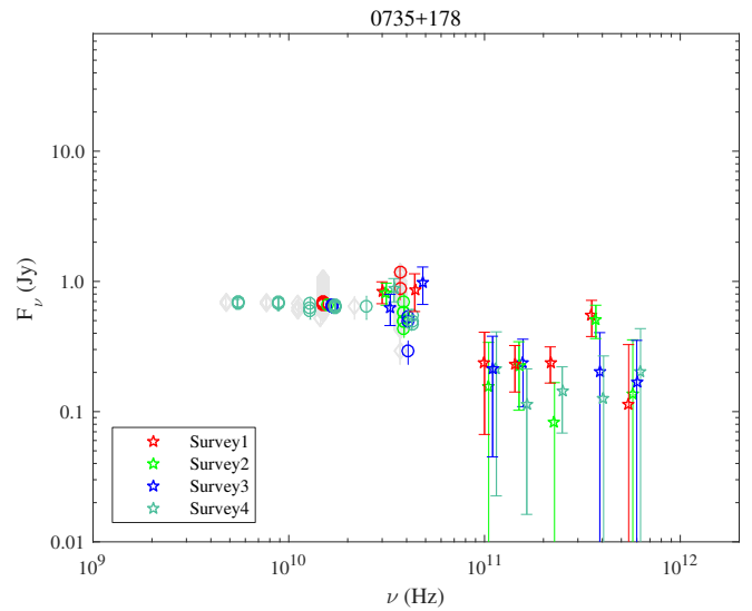
Fig. A.32. 0735+178.
