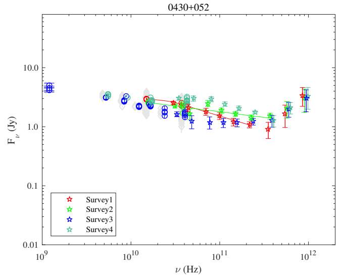
Fig. A.22. 0430+052.
