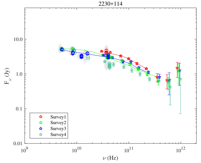
Fig. A.100. 2230+114.
