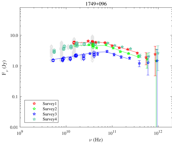
Fig. A.77. 1749+096.
