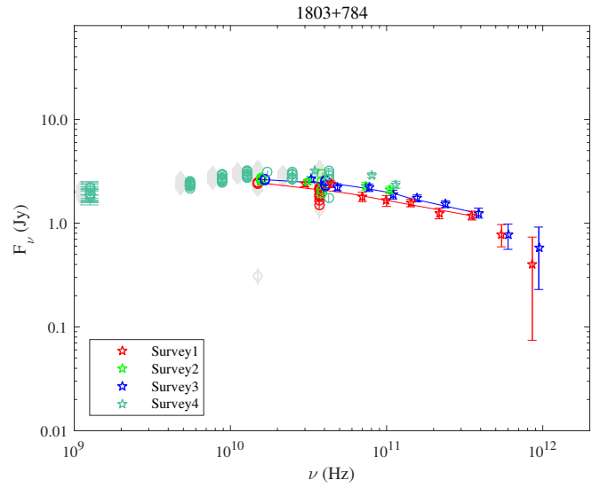
Fig. A.78. 1803+784.
