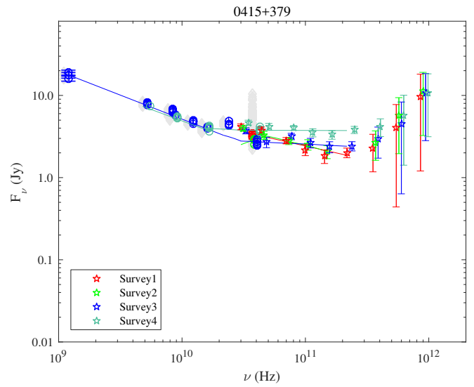
Fig. A.20. 0415+379.
