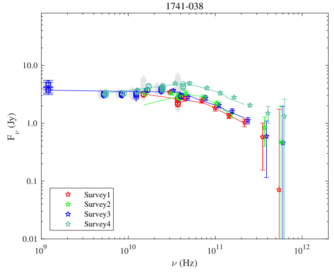
Fig. A.76. 1741-038.
