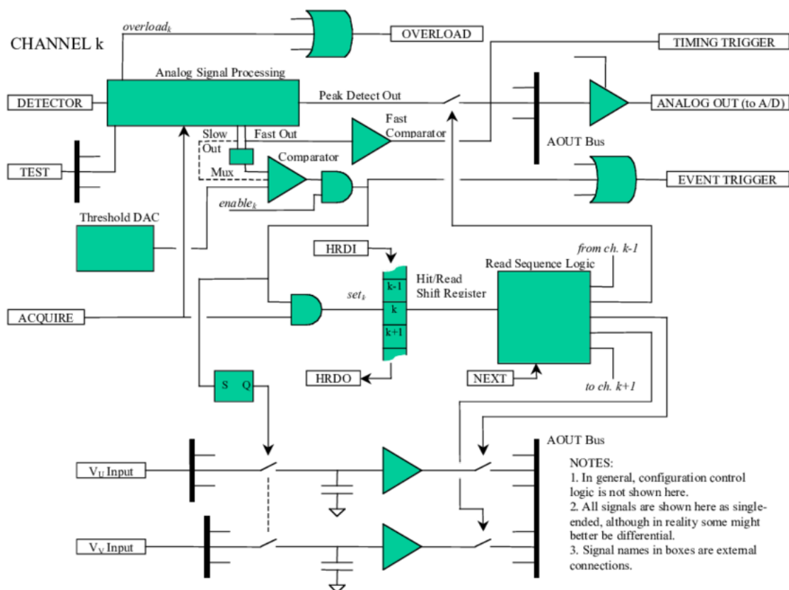
Figura 1. Schema a blocchi RENA3
