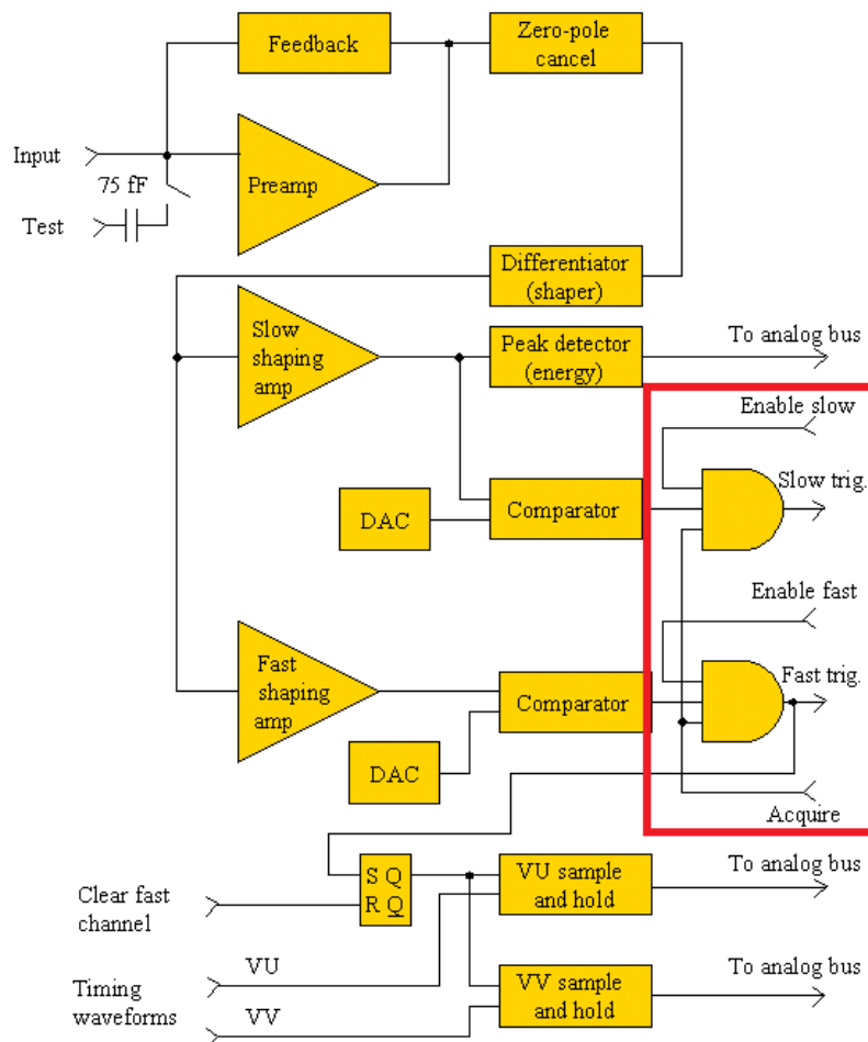
Figura 3. Schema a blocchi del singolo canale del RENA3.
