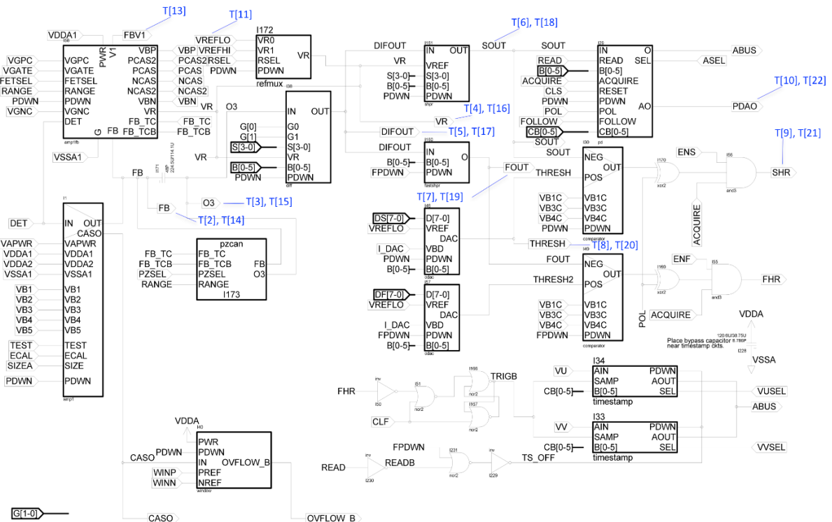
Figura 5. Schema a bocchi del singolo canale del RENA3 con relativi pin di TEST per il debug dei problemi.
