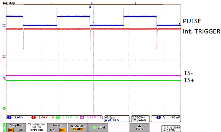
Figura 4. Impulso di test e relativi trigger interni ed esterni.
