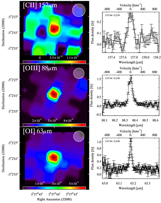
SBS0335-052
