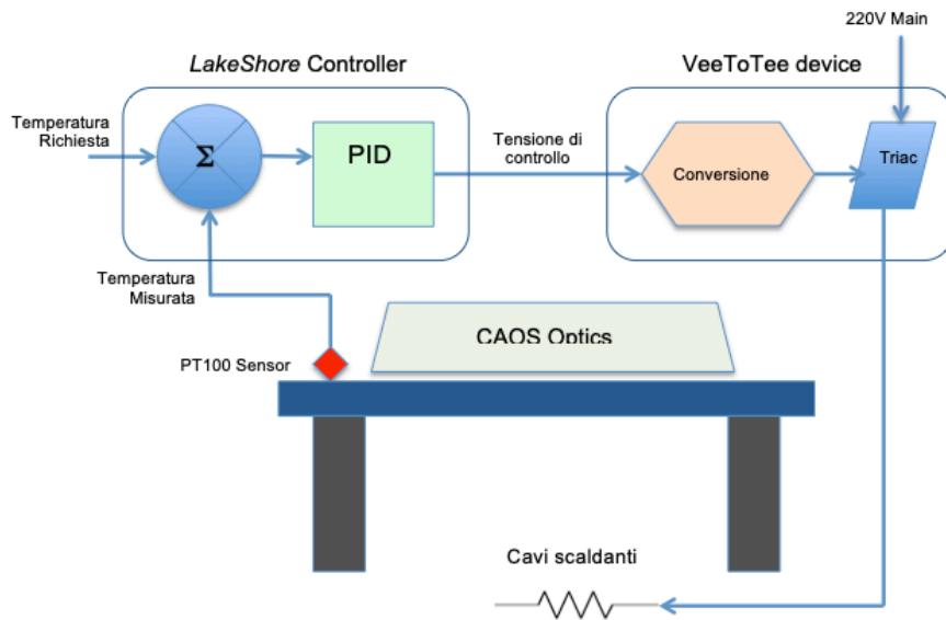
Fig. 1: CAOS – Loop di controllo della temperatura
