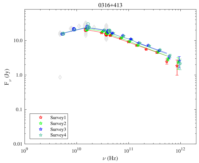
Fig. 1.16. 0316+413.
