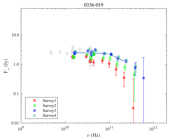
Fig. 1.18. 0336-019.
