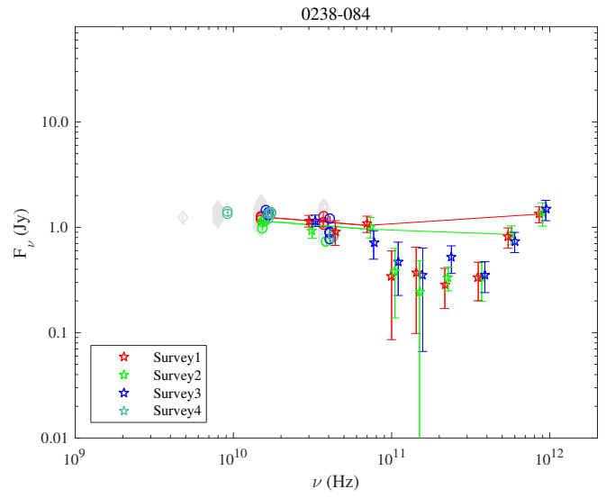
Fig. 1.14. 0238-084.
