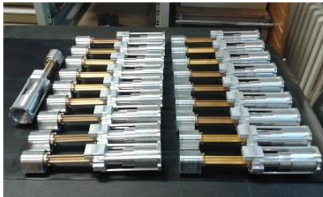
Fig. 2.1 Le 19 catene passive costituite da horn, iniettore di marca, polarizzatore, omt
