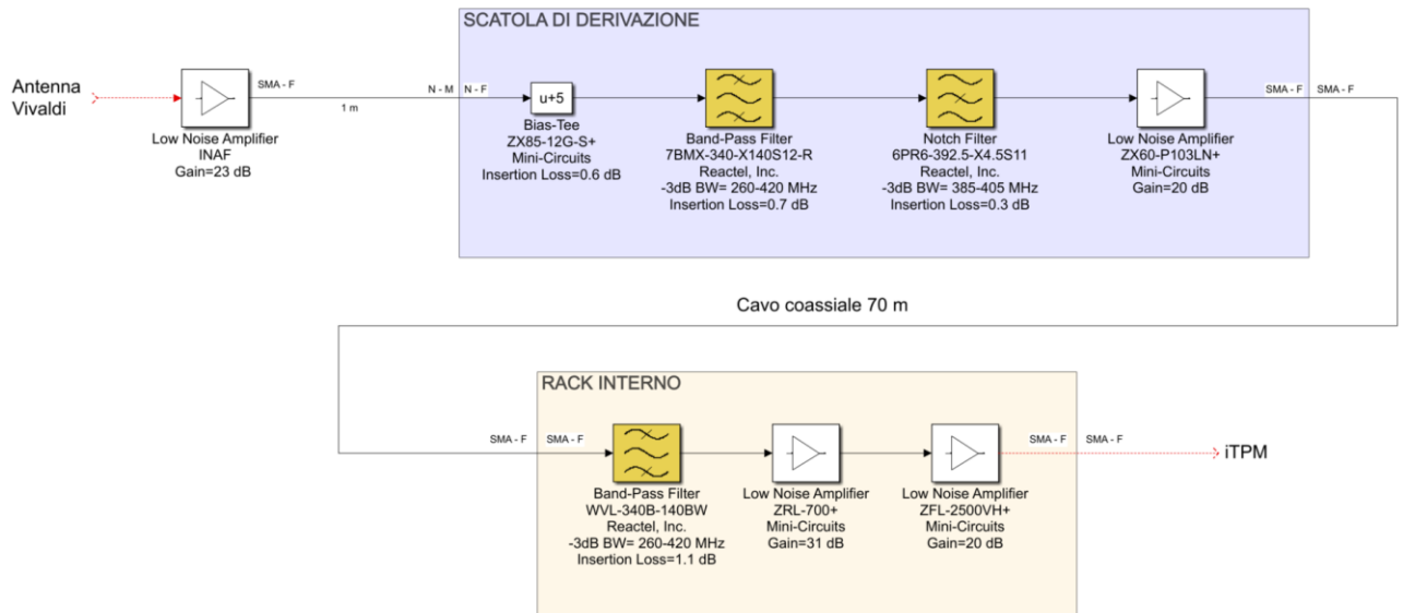
Figura 13 – Schema a blocchi della catena di acquisizione del segnale per il sistema SADino .
