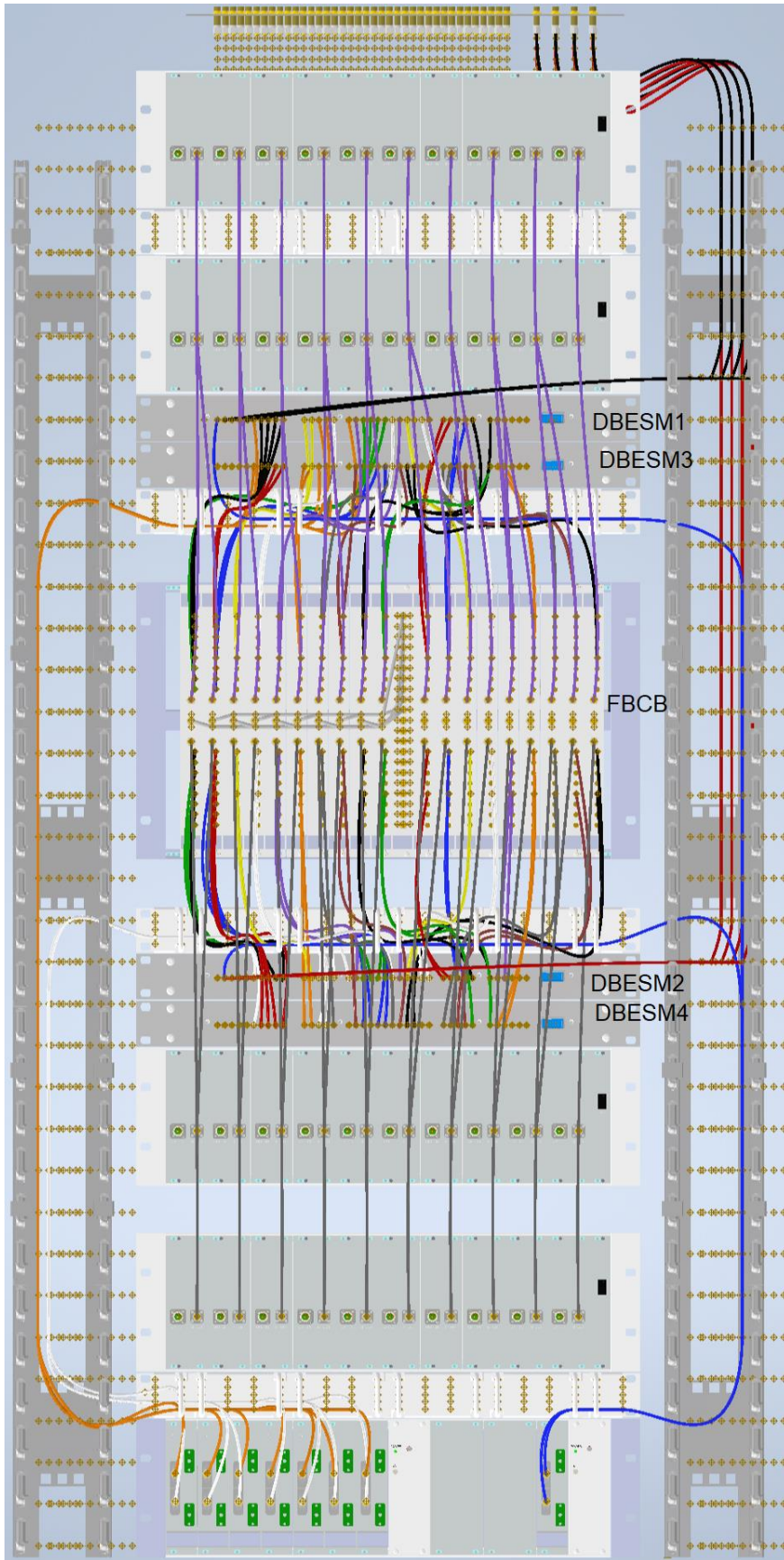
Fig 2.1 Armadio rack che ospita le pcb FBCB e DBESM
