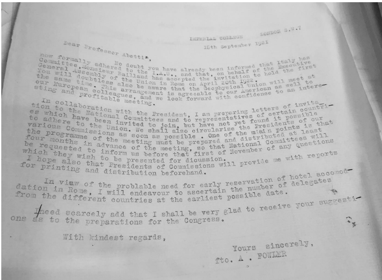
FIGURA 3: Lettera di A. Fowler ad A. Abetti, datata 16 settembre 1921, con la quale si annuncia l'adesione formale dell'Italia alla IAU (Archivio Storico Osservatorio Astronomico di Brera).
