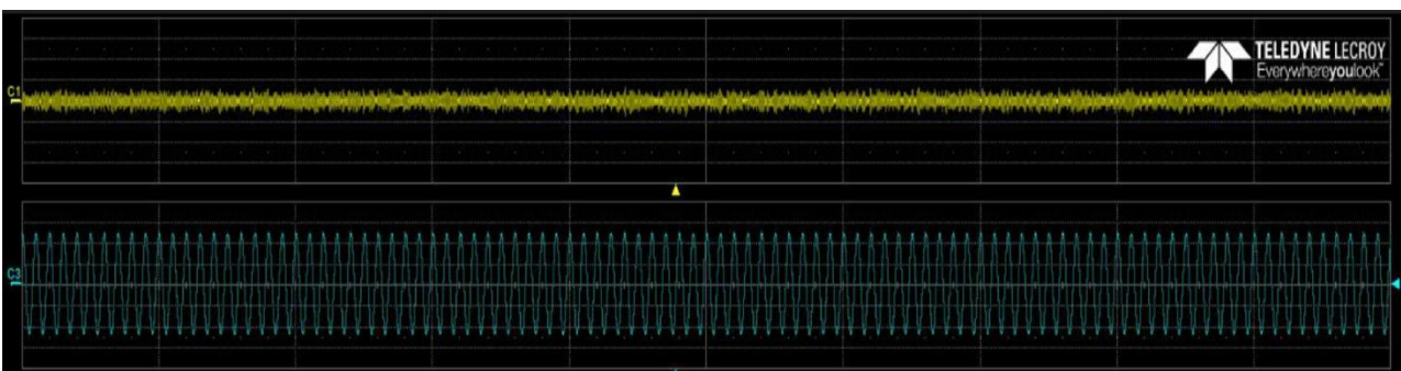
Figura 10. Ripple d'ingresso (blu) e d'uscita (giallo) del regolatore.
