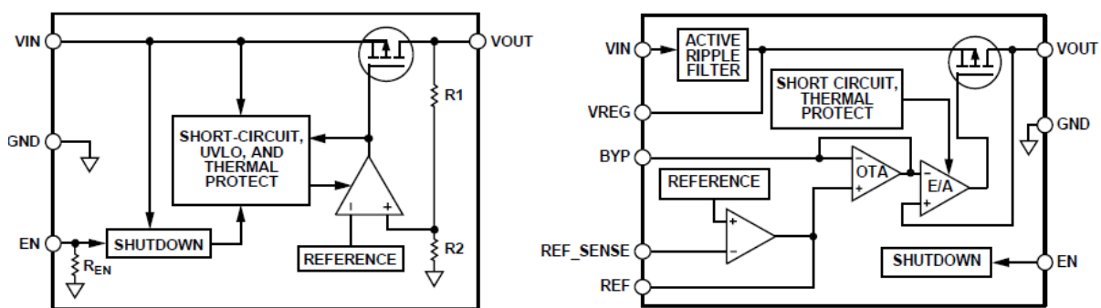
Figura 14. A sinistra lo schema a blocchi dell'ADP151 mentre a destra quello dell'ADM7150.
