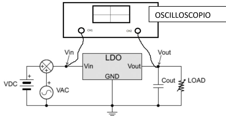
Figura 1. Metodo di misura del PSRR
