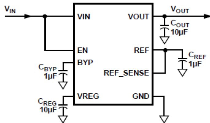
Figura 16. Schema elettrico AMD7150
