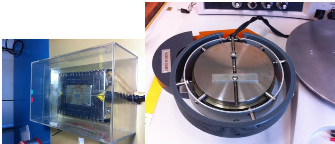
Figura7 Sistemi adottati di essicazione e polimerizzazione dell'adesivo. A sinistra fornello flussato in N. A destra piastra termica a temperatura controllata.
