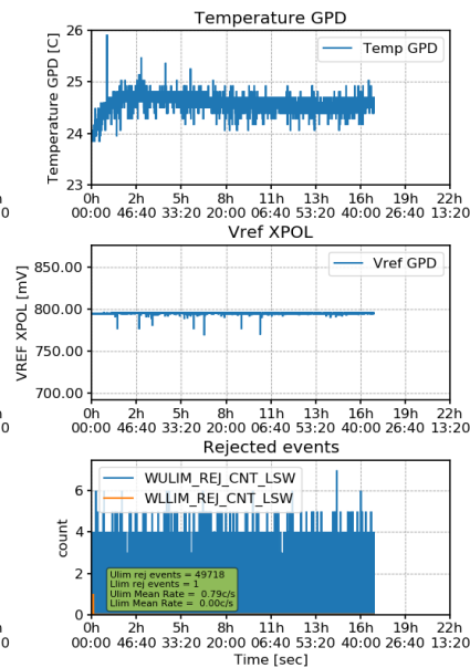
DU 2[FM2] - Analog HK - 20143 2019-10-23 15:16:39 - 2019-10-24 08:47:04
