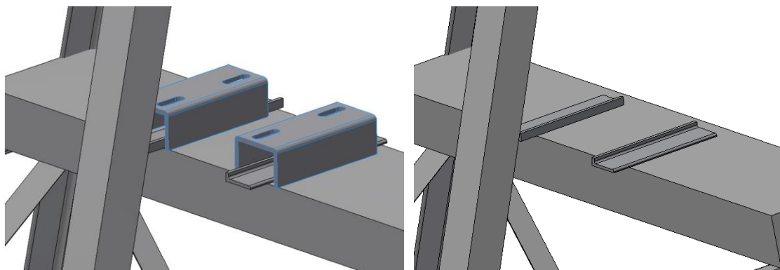
Figura 6: Rimozione vecchi supporti
