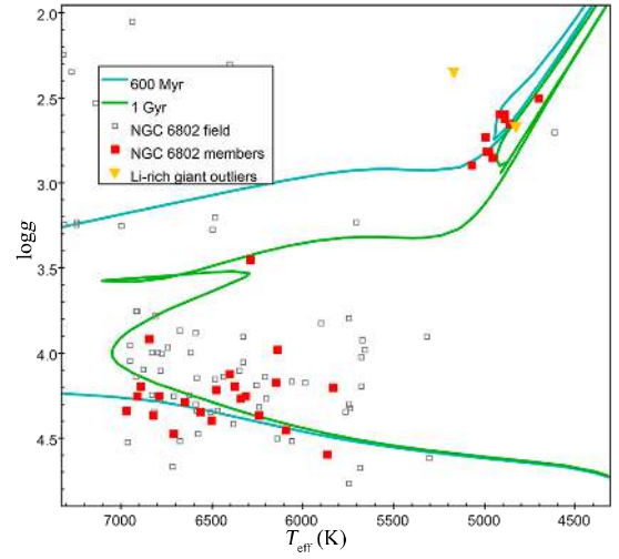
Fig. B.189. Kiel diagram for NGC 6802.
