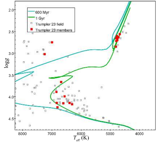
Fig. B.171. Kiel diagram for Trumpler 23.
