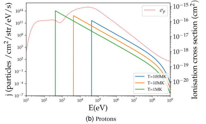
(b) Protons
